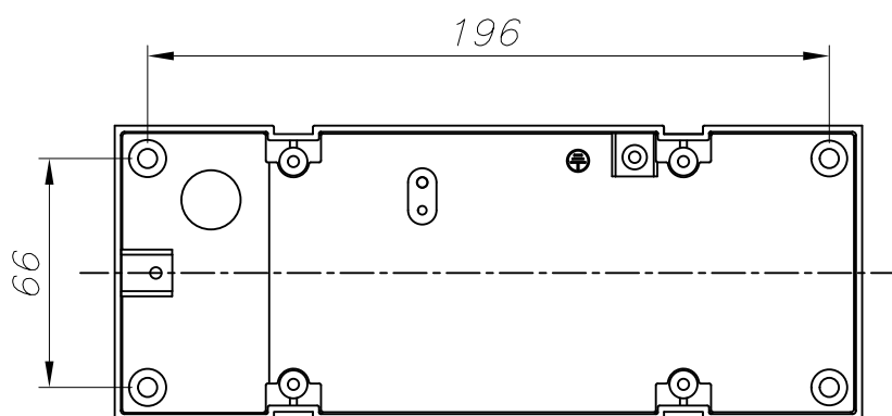
PLANTILLA DE INSTALACIÓN INSTALLATION TEMPLATE
