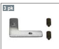
Skjøt 90° utside Art. nr: 314265300 Farge: Alu
