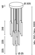
13x3W / 2194lm / 2700K / CRI 80
