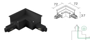
L Connector - Inside Kan tilkobles strøm
