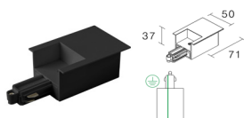
End Feed - Left Kan tilkobles strøm
