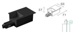
End Feed - Right Kan tilkobles strøm
